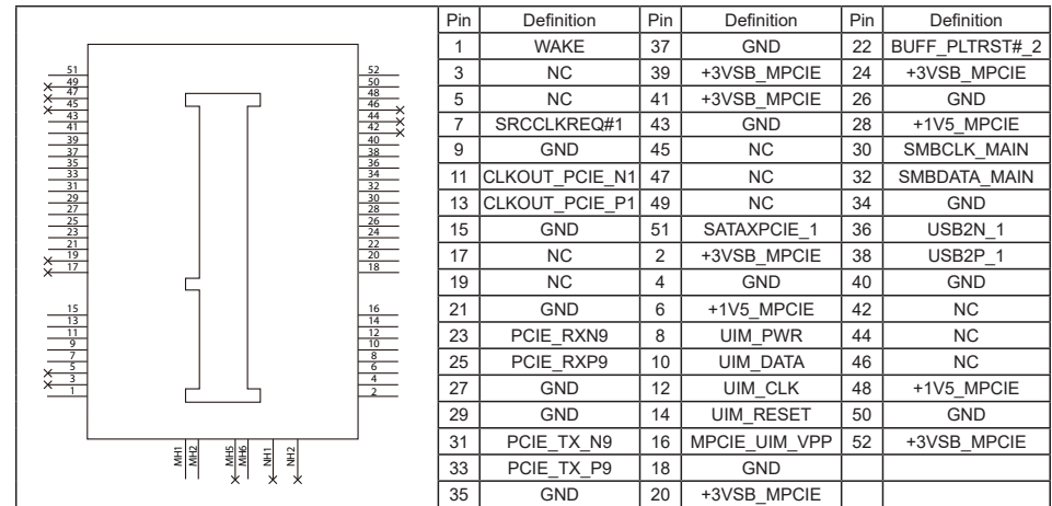
MPCIE1: mini-PCIe Slot
