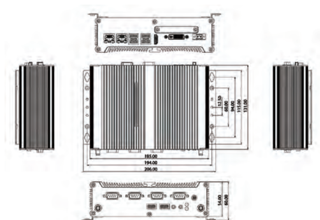
NISE104 寸法図 (単位: mm)
