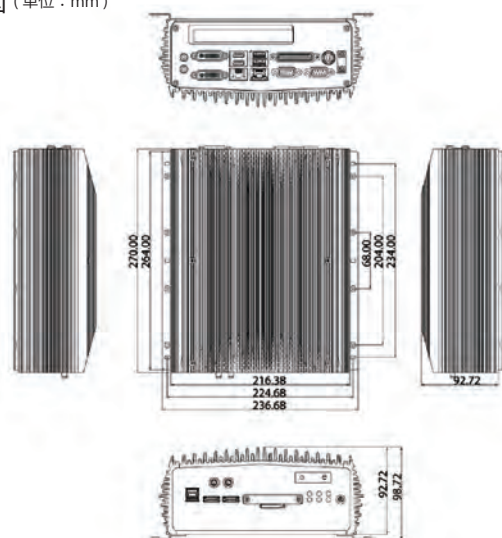
NISE3600 寸法図 (単位: mm)
